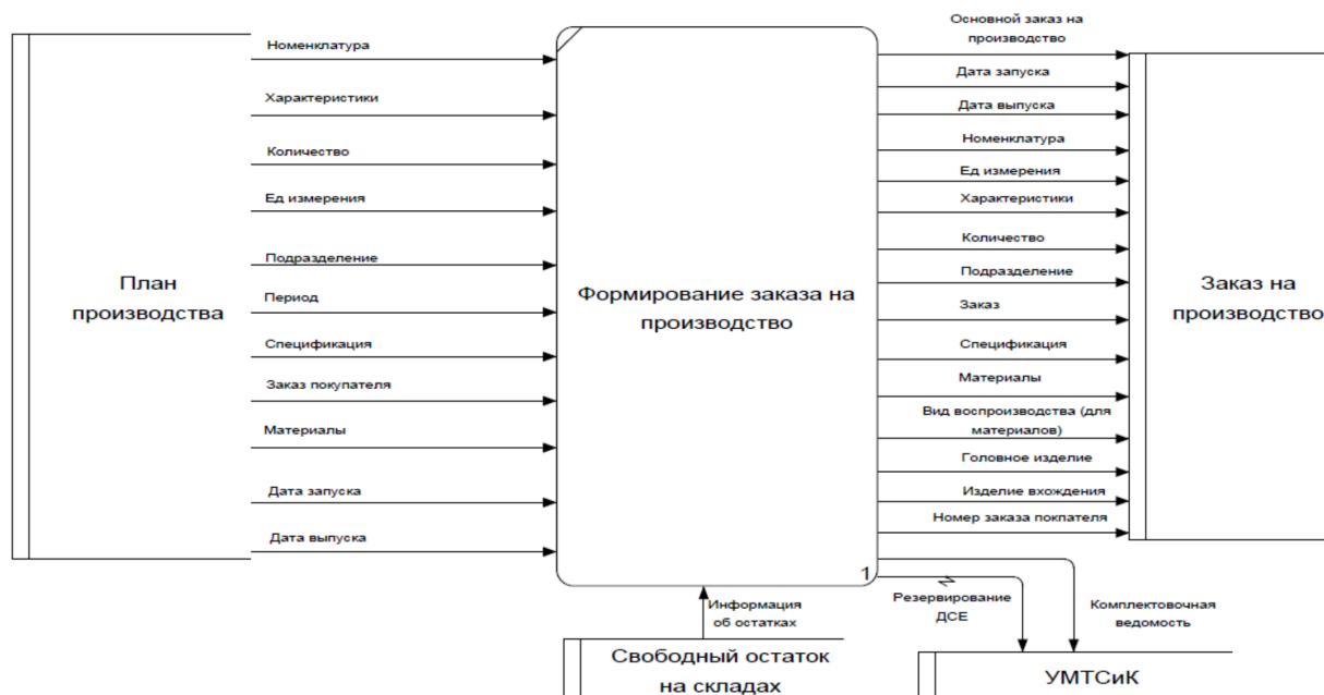
Диаграмма 2 – Формирование заказа на производство
