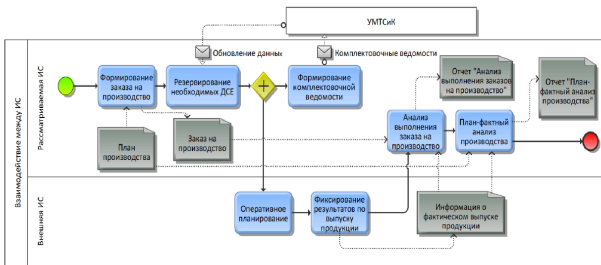
Диаграмма 2 – Взаимодействие между ИС
